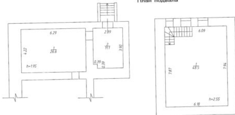
План подвала
